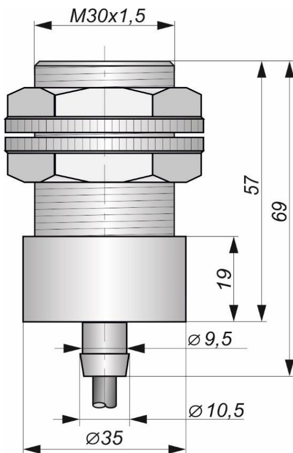
Габаритный чертеж
